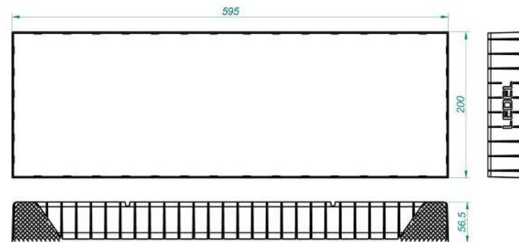
Рисунок 1а Светильники «L-school 16»
